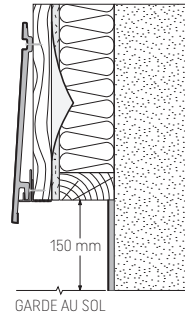
FS-262 Profil de ventilation, clipsable
