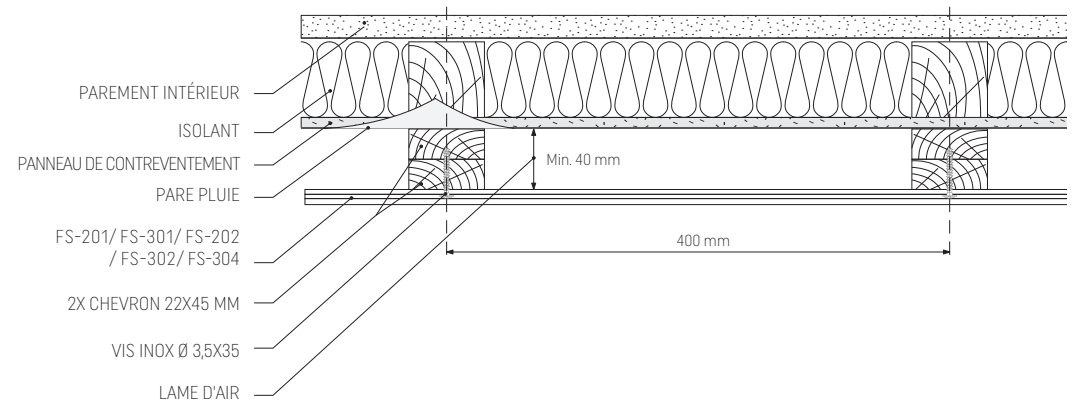
Fig. 9. Lame d'air de 40 mm - coupe horizontale, voir page 8
