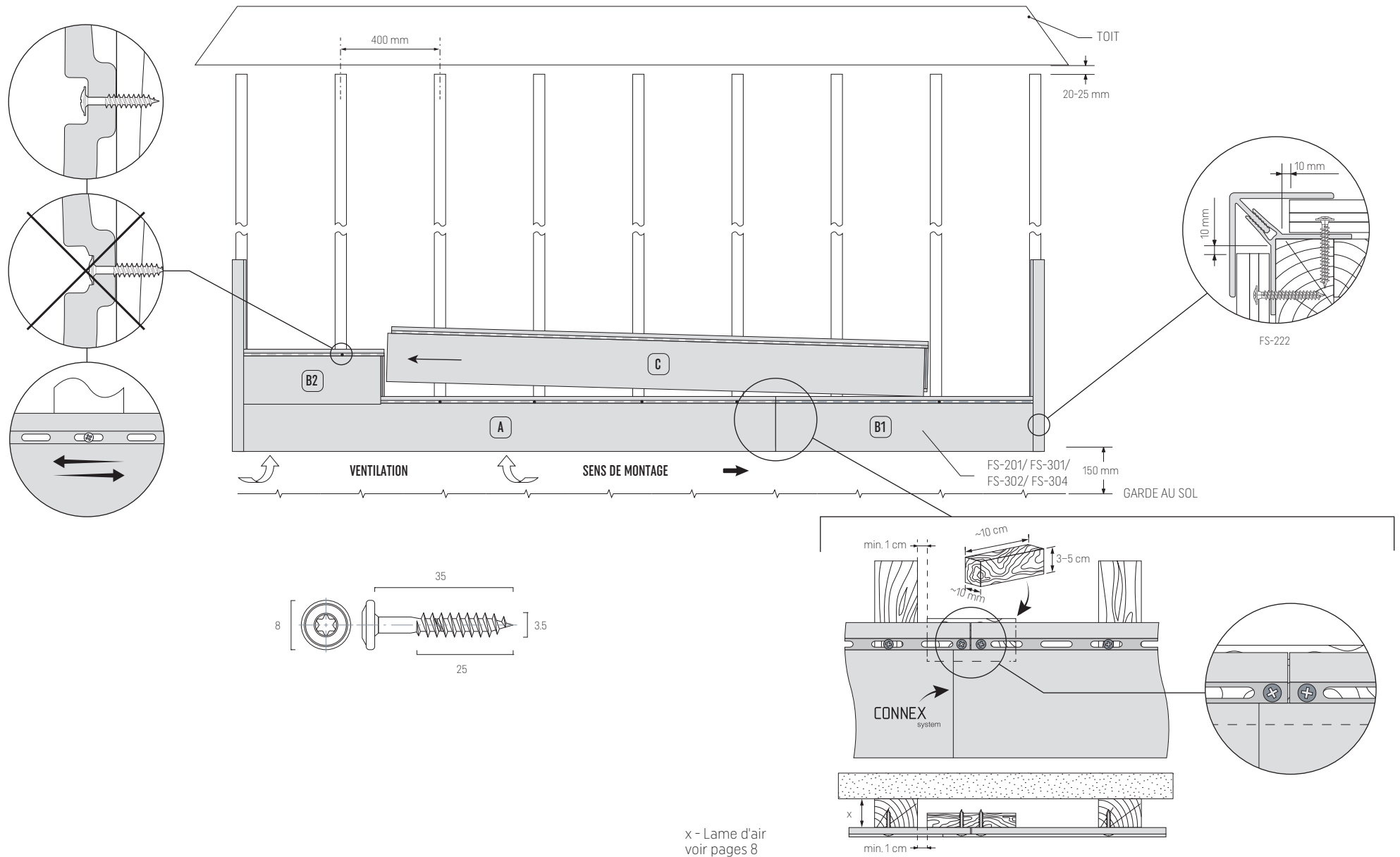
Fig. 5. Règles pour assembler les lames de bardage (FS-201/ FS-301/ FS-302/ FS-304) - le système CONNEX, 2,95 ml
