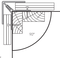
FS-222 Profil d'angle, universel, clipsable
