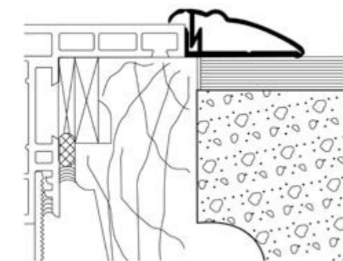
MGR3514 en application
