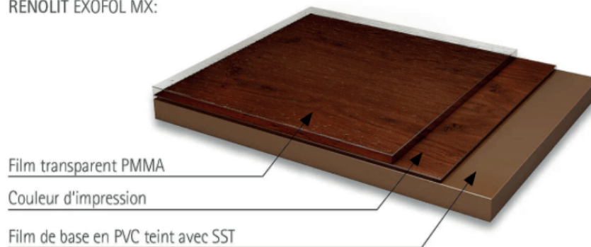
Structure schématique de la feuille extérieure RENOLIT EXOFOL MX:
