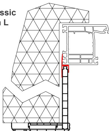
Ebrasement avec planche alvéolaire
