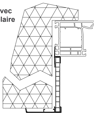
Départ sur dormant à aile de guidage
